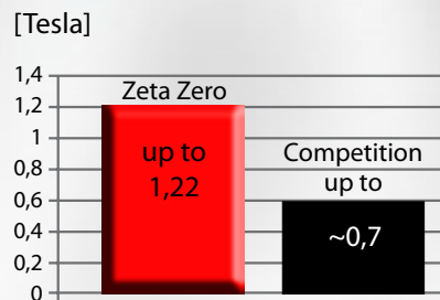
Indukcja w szczelinie i siła pola magnetycznego Gap Flux & Force [Tesla]
